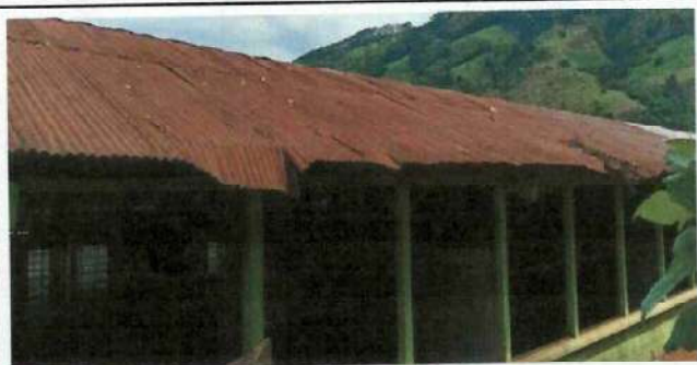
Foto 1: Se observa el deterioro de lámina de la estructura portante de tres aulas y dos bodegas
